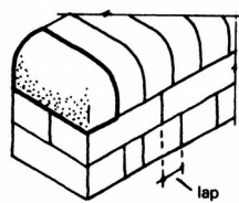
⑦ Bull nose return on edge
